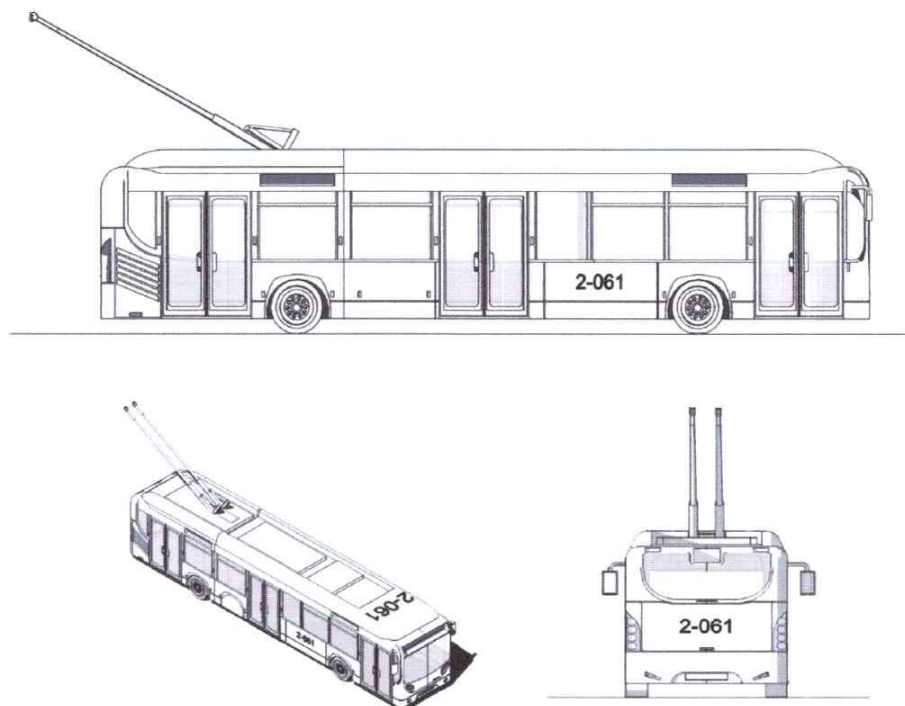
Зураг 13. Троллейбусны гараашны дугаар (Жишээ зураг)
