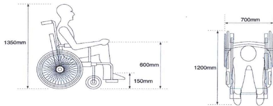
Зураг 8. Тулгуур эрхтний хөгжлийн бэрхшээлтэй иргэн тэргэнцэртэй зорчих зай (Жишээ зураг)
