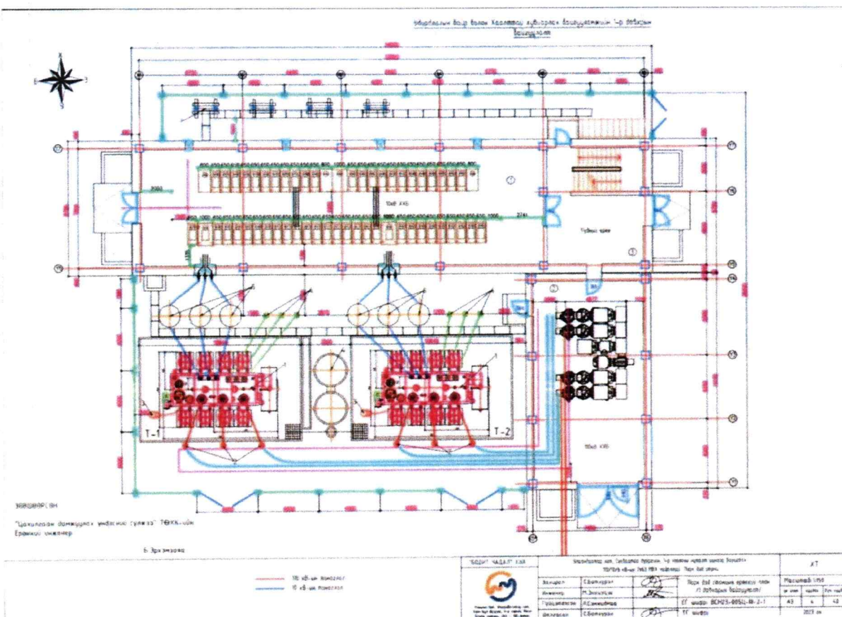
Зураг 1. 110/10 кВ-ын 2х63 МВА чадалтай “Парк” дэд станцын Удирдлагын байр болон Хаалттай хуваарилах байгууламжийн төлөвлөлт
